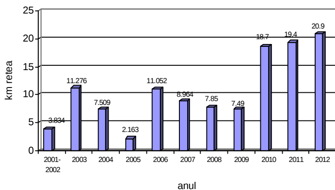
Extinderi retele de canalizare in perioada 2001-2012
